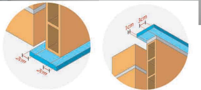
Detalle ESV-02.c-R4
