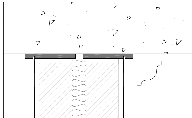
Detalle ESV-02.a.R5
