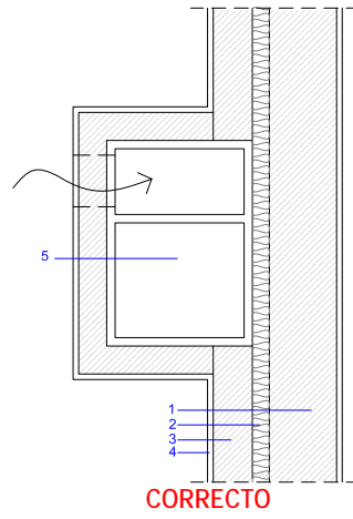
ESV-02.b-Ci6
