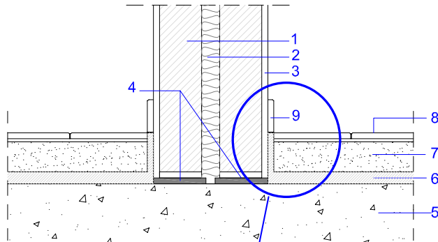
Detalle ESV-02.a-Fo1
