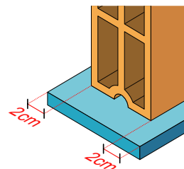
Detalle ESV-02.b-R4
