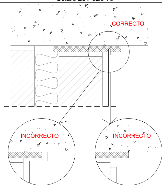
Detalle ESV-02.c-V6
