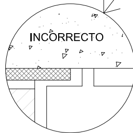
Detalle ESV-02.a.V4
