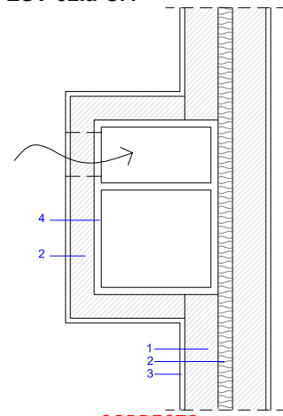
ESV-02.a-Ci4
