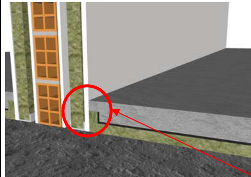
Detalle SF-01.a.V1
