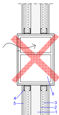
ESV-01.a.b-Ci3 PLANTA
