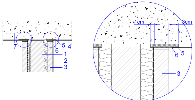
Detalle ESV-02.c.R2
