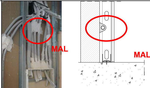
Detalle ESV-01.a.V2
