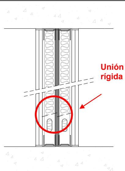
Detalle ESV-03.a.V1
