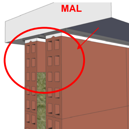
Detalle ESV-02.a.V5
