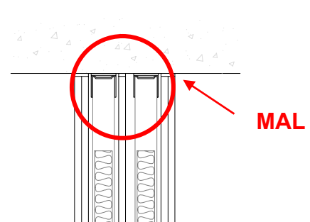
Detalle ESV-03.a.V2
